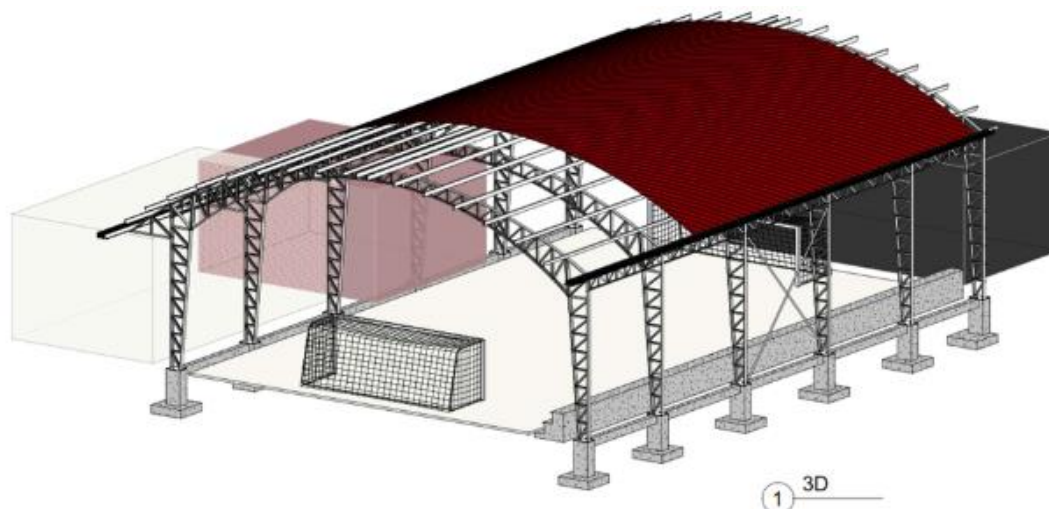
Foto 32: Estudio para la construcción de la cubierta metálica - Modelo 3D. Octubre 2023.
